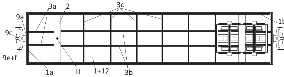
Schemat montażu wręgów
